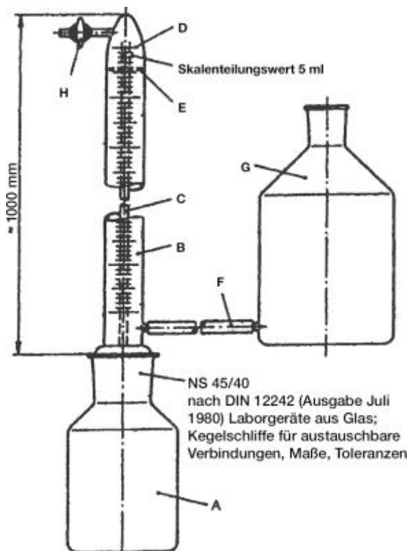
Bild 2: Versuchsapparatur zur Bestimmung des Faulverhaltens von Schlamm nach DIN 38414-8, Seite 6, Ausgabe Juni 1985
